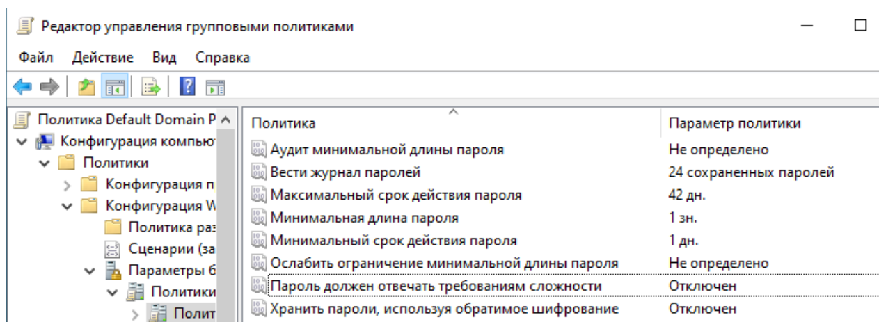
рисунок 6 - измененная групповая политика паролей
